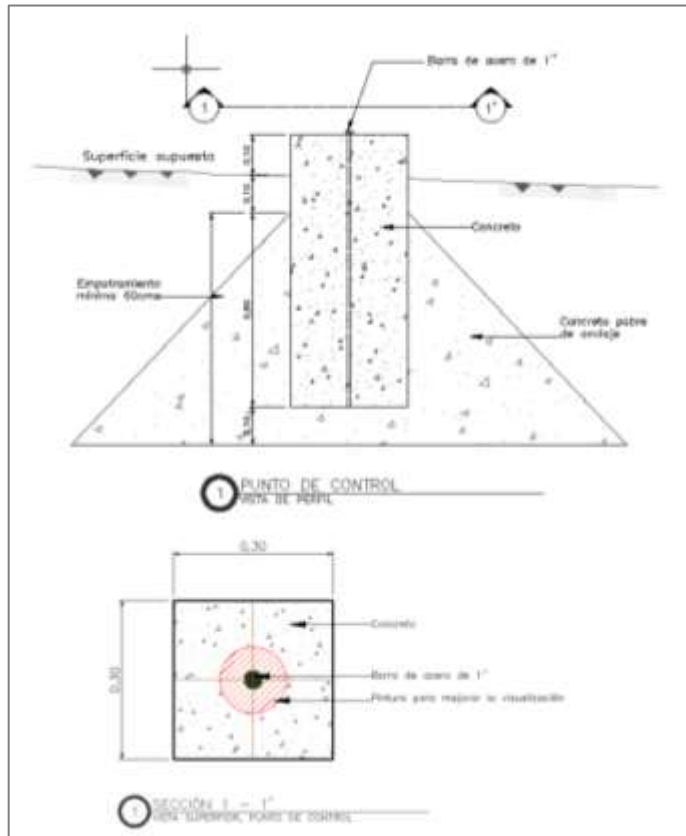
Figura 8.2 Punto de control, vista de perfil y superior.
