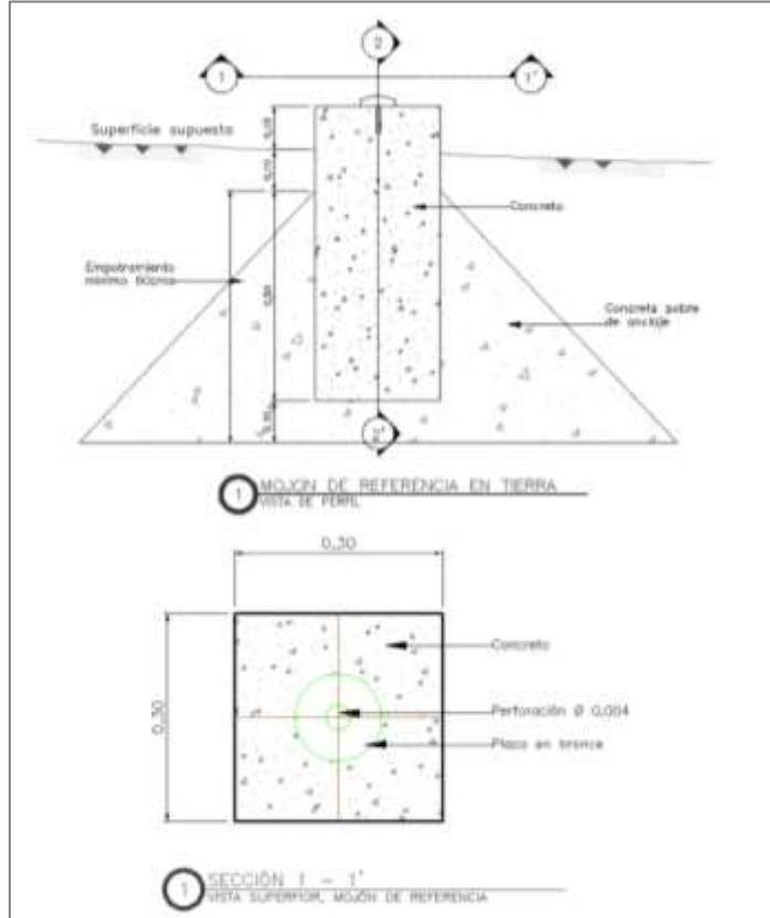
Figura 8.1 Mojones de referencia en tierra, vista de perfil y superior.
